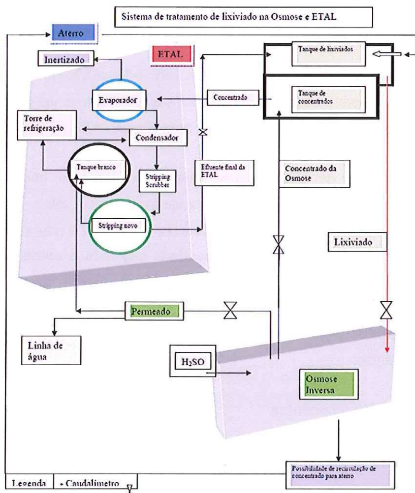
Figura 9 - Esquema do sistema de tratamento de lixiviados
